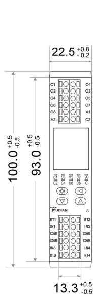
主视图
