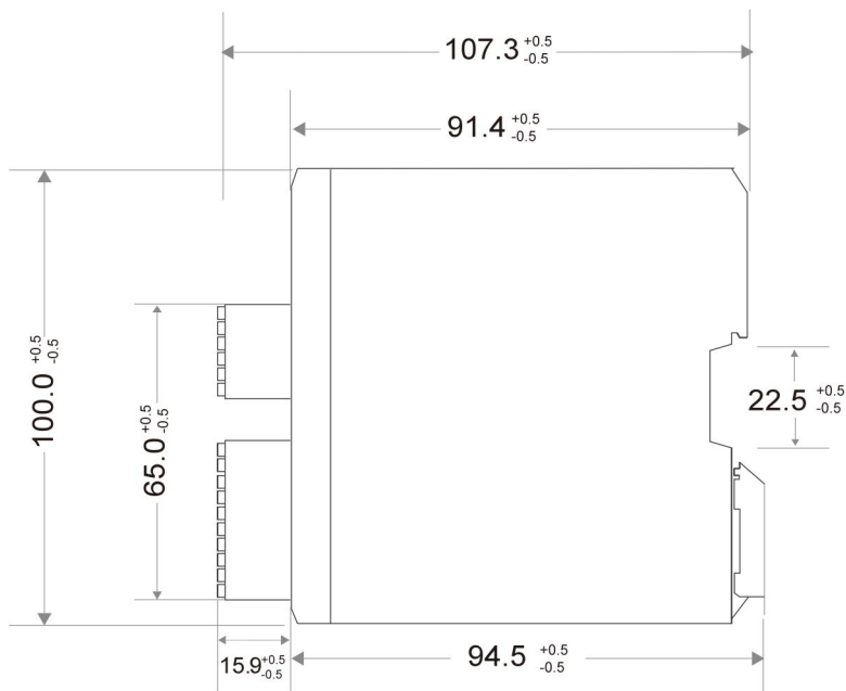
侧视图
